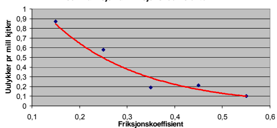
Ulykkesfrekvens (personskadeulykker pr mill. kjøtkm) som funksjon av friksjonskoeffisienten
